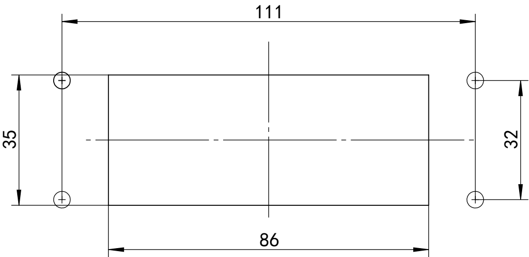
面板开孔图
