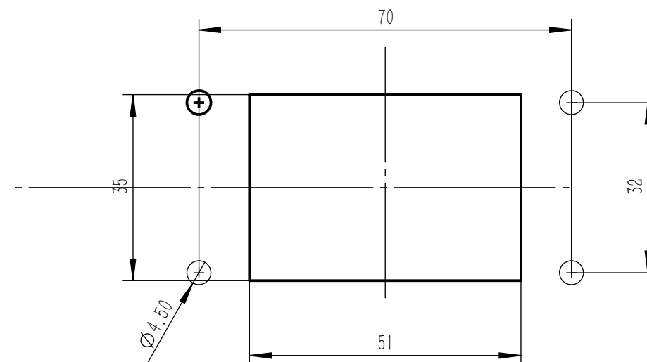
面板开孔图
