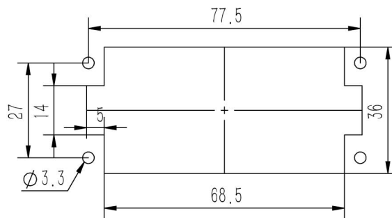
面板开孔图
