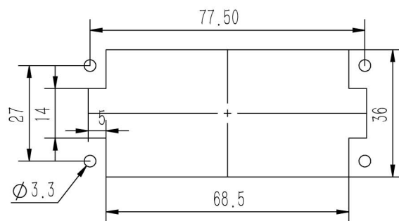
面板开孔图
